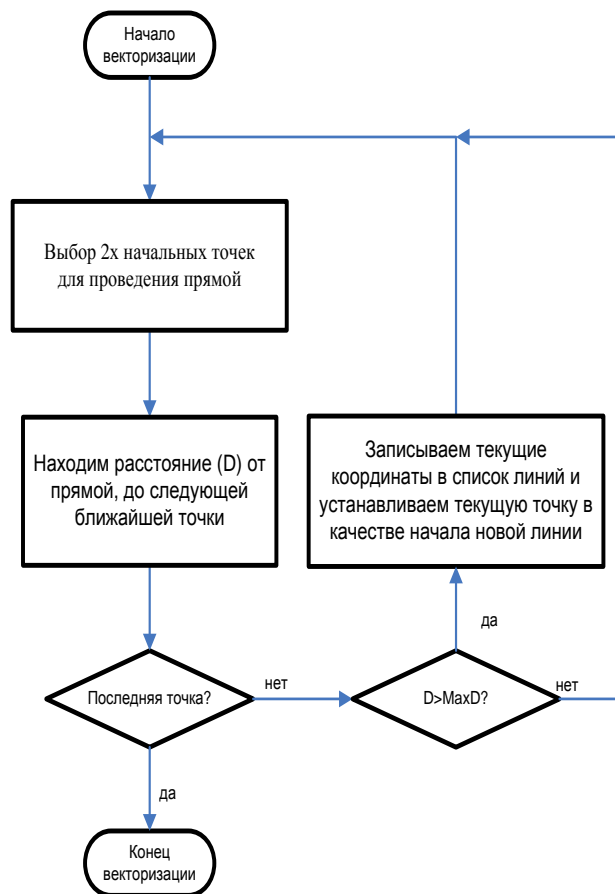
Алгоритм векторизации тонкого контура.
