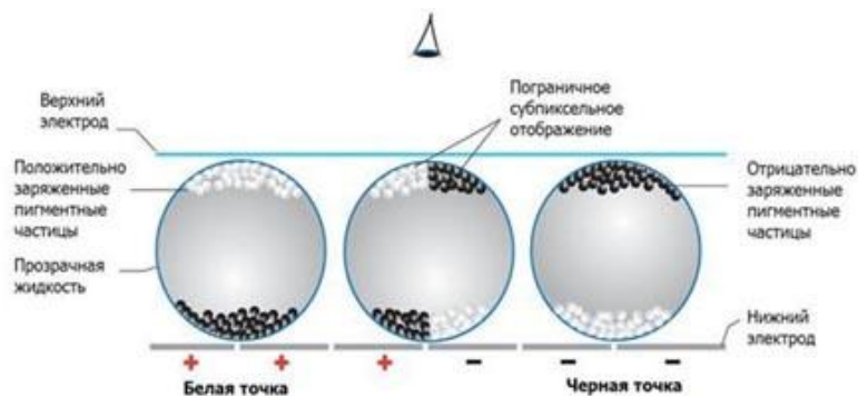
Микрокапсулы электронных чернил.
