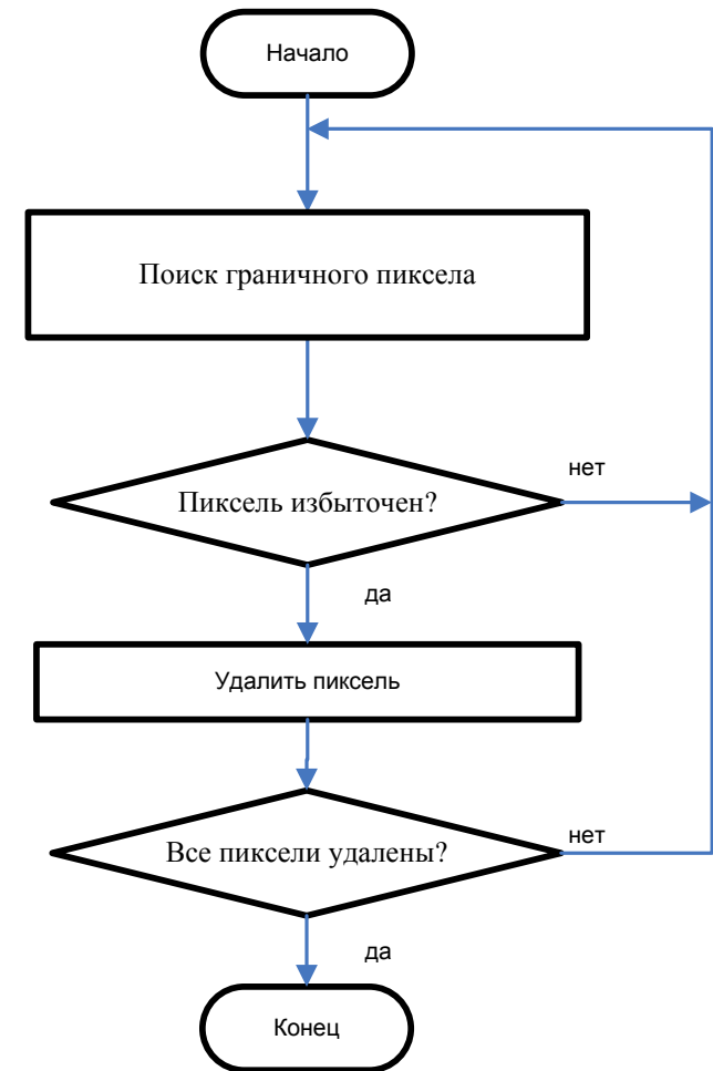
Алгоритм составления тонкого контура
