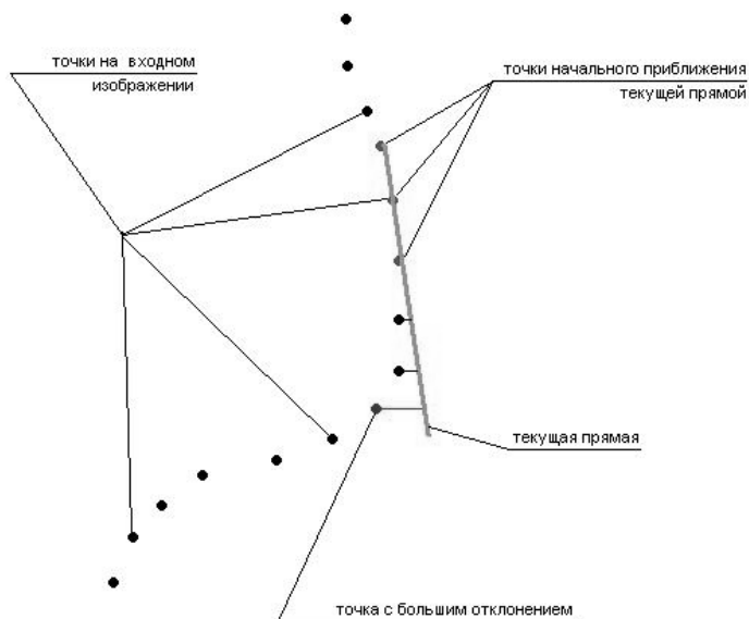
Метод последовательных приближений.
