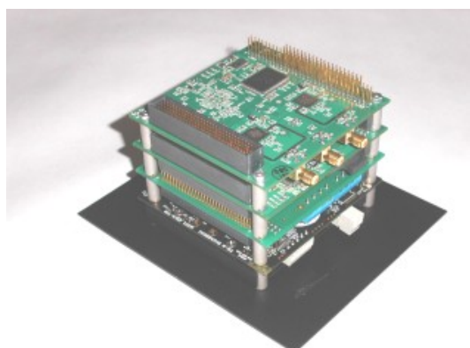
Управляющий блок в стандарте PC-104+
