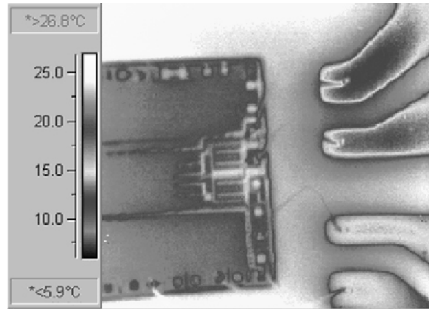
Рис. 3. Изображение микросхемы, полученное с помощью тепловизора ThermoCAM фирмы FLIR и показывающее проводники размером 7 мкм [3]
