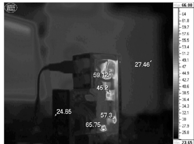
Рис.1. Тепловое поле блока питания монитора
