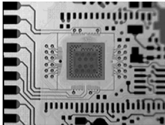
Рис. 4. ИК-камера в сочетании с микроскопом становится ИК-микроскопом, способным исследовать объекты размером 5 мкм [3]
