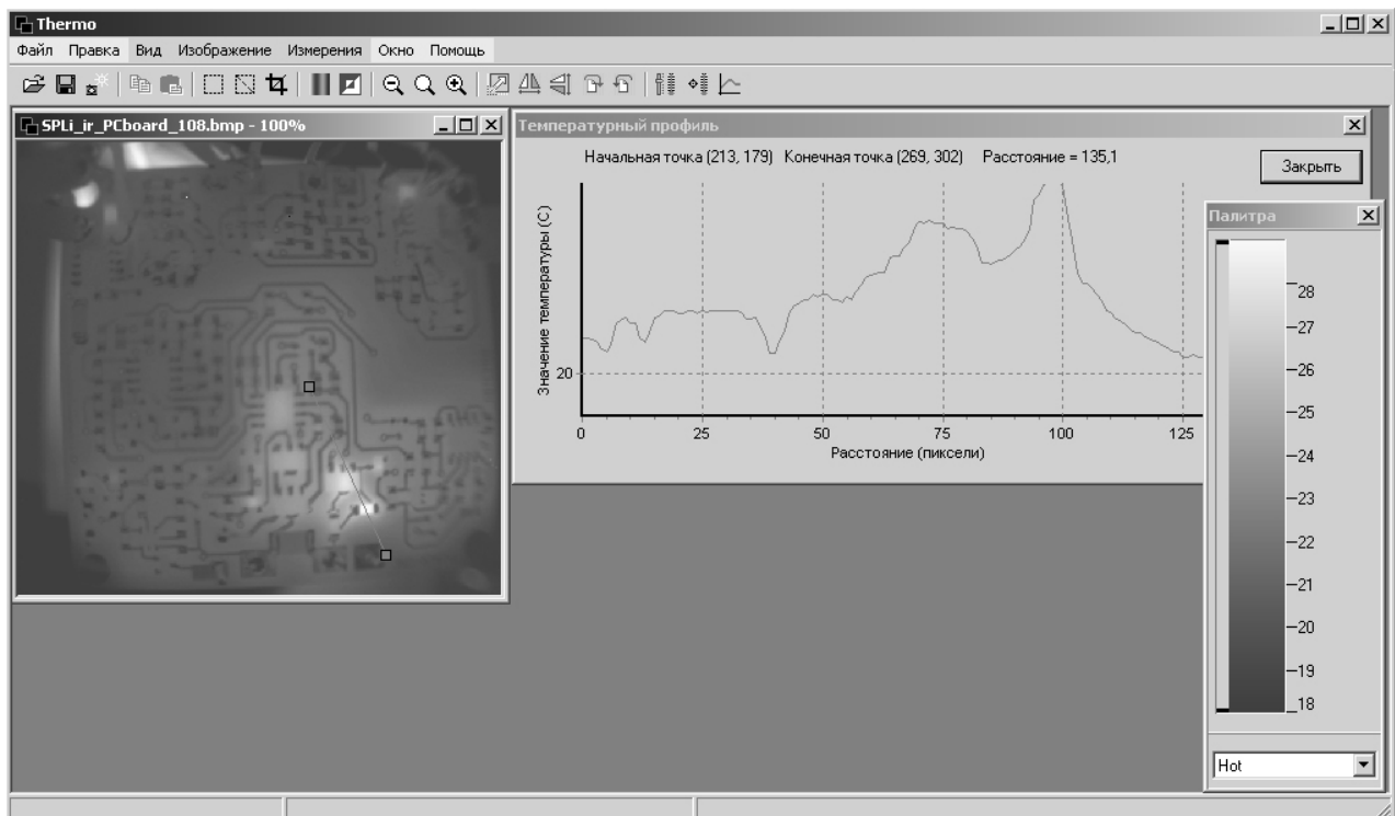
Рис. 6. Окно программы Thermo (разработка кафедры ИУ4 «Проектирование и технология производства электронно-вычислительных средств» МГТУ им. Н. Э. Баумана) с температурным профилем, построенным для критического участка печатной платы
