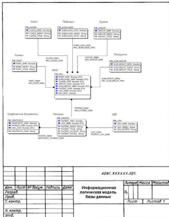
Рисунок 5.5 - Пример оформления информационной логической модели конструкторско-технологической базы данных (IDEF1X)
