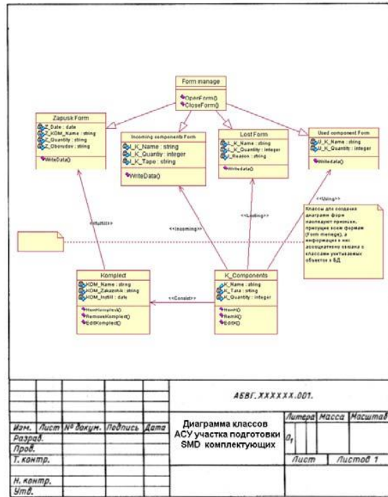
Рисунок 5.7 - Пример оформления объектной модели (диаграмма классов)
