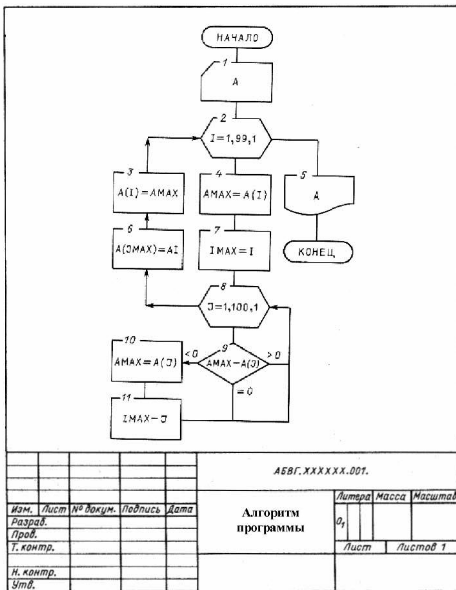
Рисунок 5.2 - Пример оформления алгоритма программы
