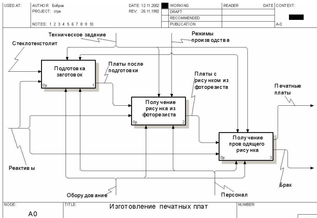
Рисунок 5.3 - Пример оформления структурно-функциональной модели технологического процесса (IDEF0)
