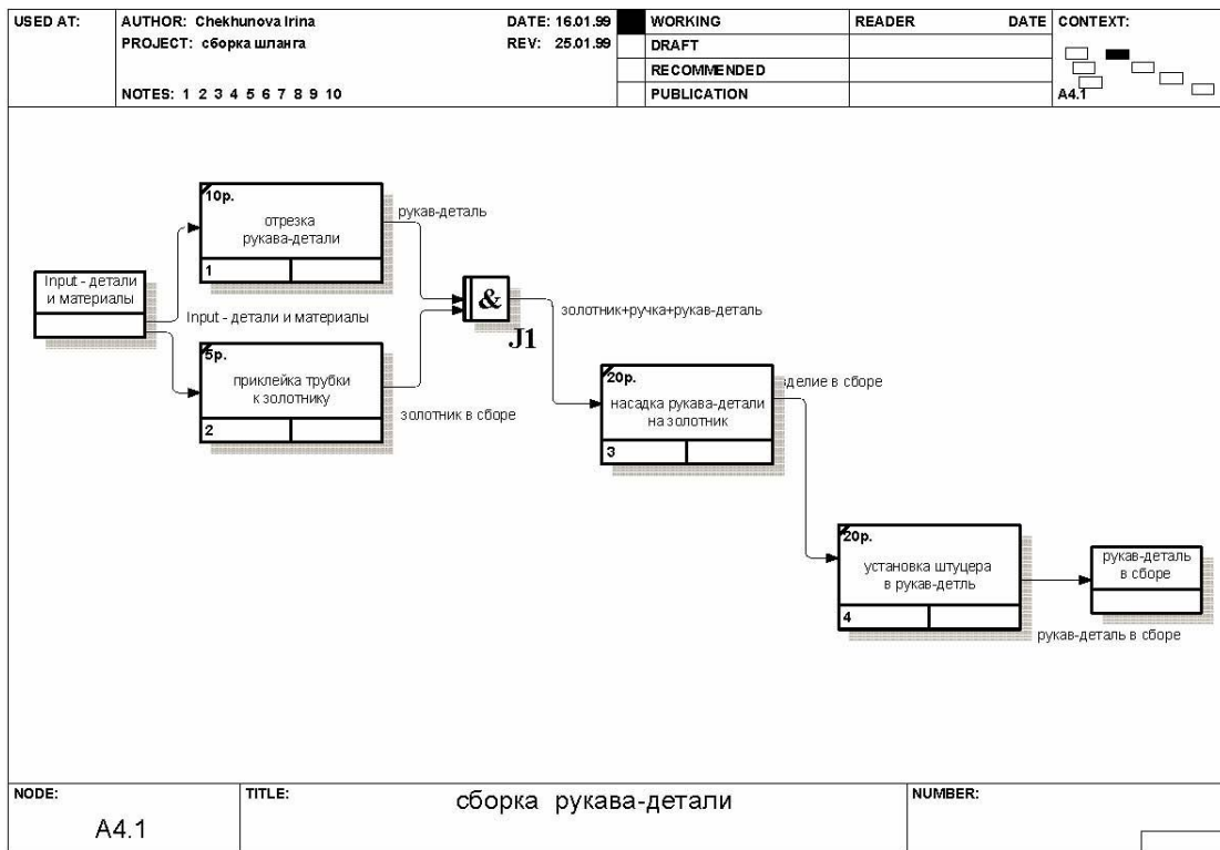
Рисунок 5.4 - Пример оформления структурно-функциональной модели технологического Процесса (IDEF3)
