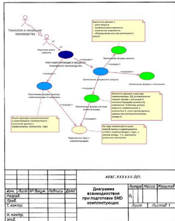
Рисунок 5.6 - Пример оформления объектной модели (диаграмма вариантов использования - Use Case)
