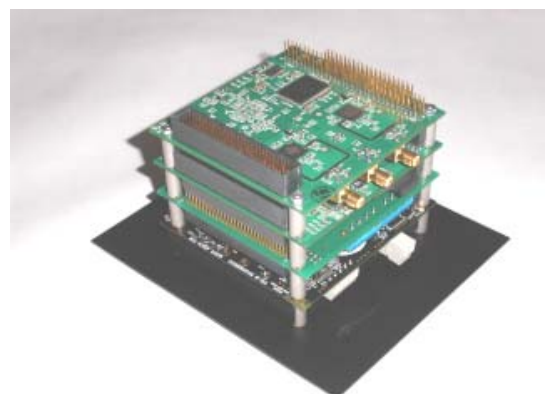
Управляющий блок в стандарте PC-104+
